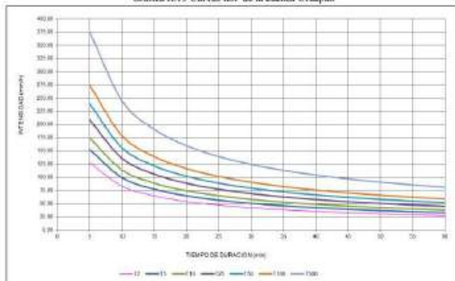
Gráfica II.15 Curvas IDF de la cuenca Uruapan
