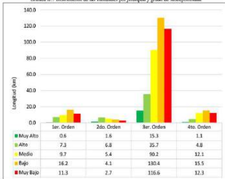
Gráfica II.7 Distribución de las vialidades por jerarquía y grado de susceptibilidad
