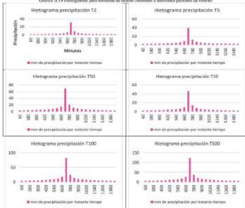
Gráfica II.14 Hietogramas para tormenta de diseño conforme a diferentes periodos de retorno
