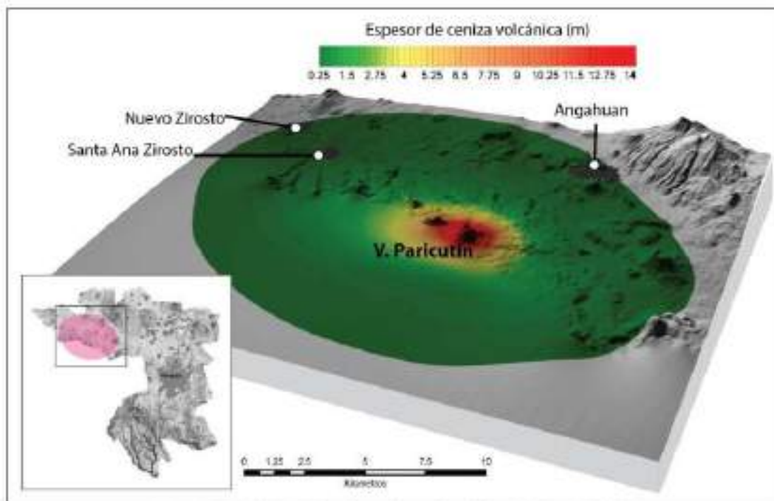
Figura II.6 Dispersión de ceniza volcánica a partir del ciclo eruptivo del volcán Parícutín
