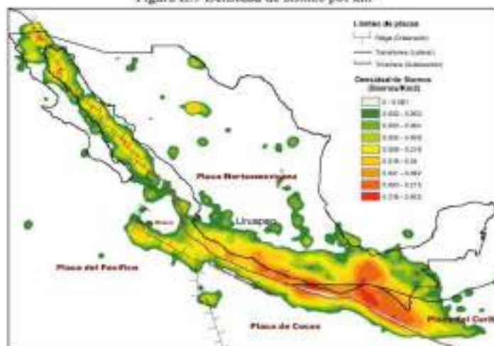
Figura II.9 Densidad de sismos por km 2
