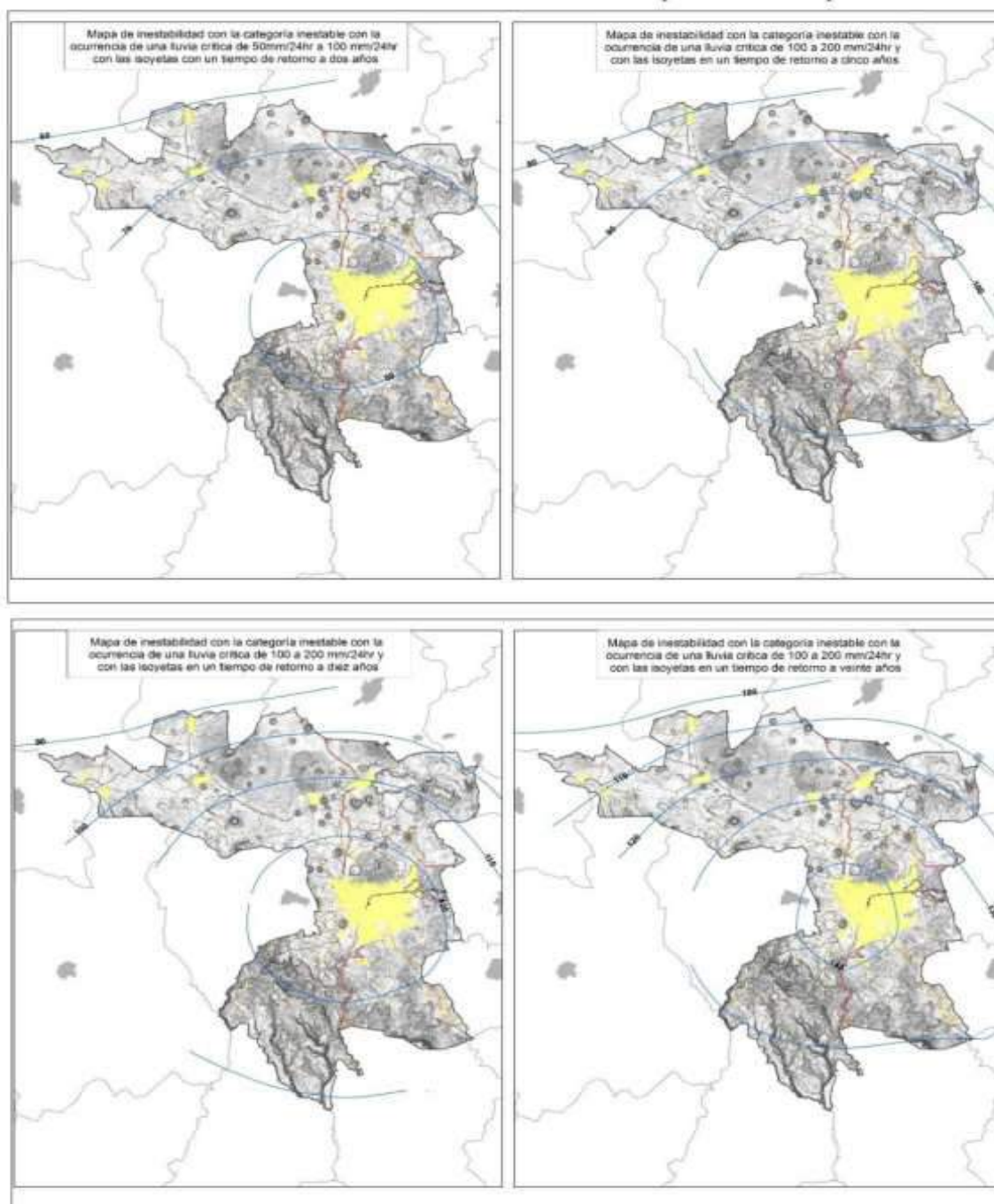
Figura II.17 Inestabilidad de laderas con diferentes lluvias críticas para diferentes periodos de retorno
