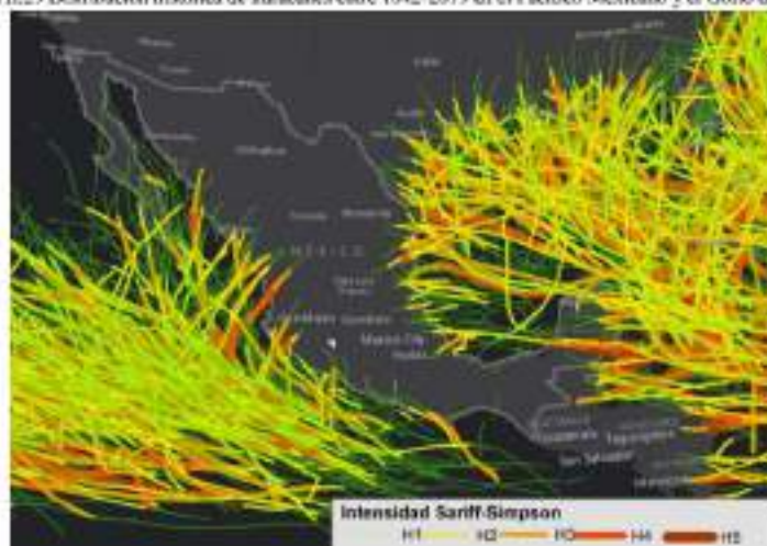
Figura II.29 Distribución histórica de huracanes entre 1842-2019 en el Pacífico Mexicano y el Golfo de México
