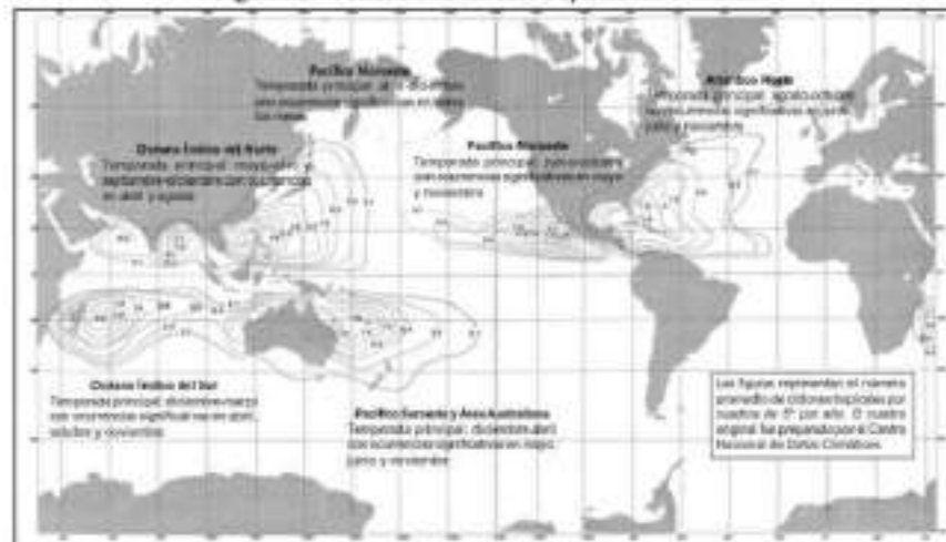
Figura II.27 Presencia de ciclones tropicales en el mundo
