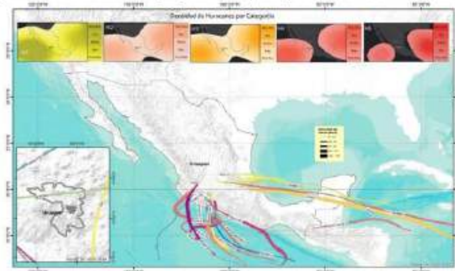
Figura II.31 Densidad de huracanes y trayectorias de aquellos que cruzaron en las cercanías de Uruapan
