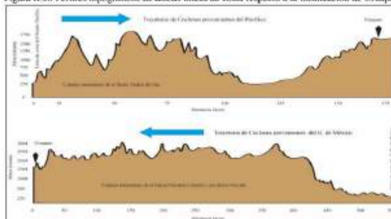
Figura II.28 Perfiles topográficos de ambas líneas de costa respecto a la localización de Uruapan
