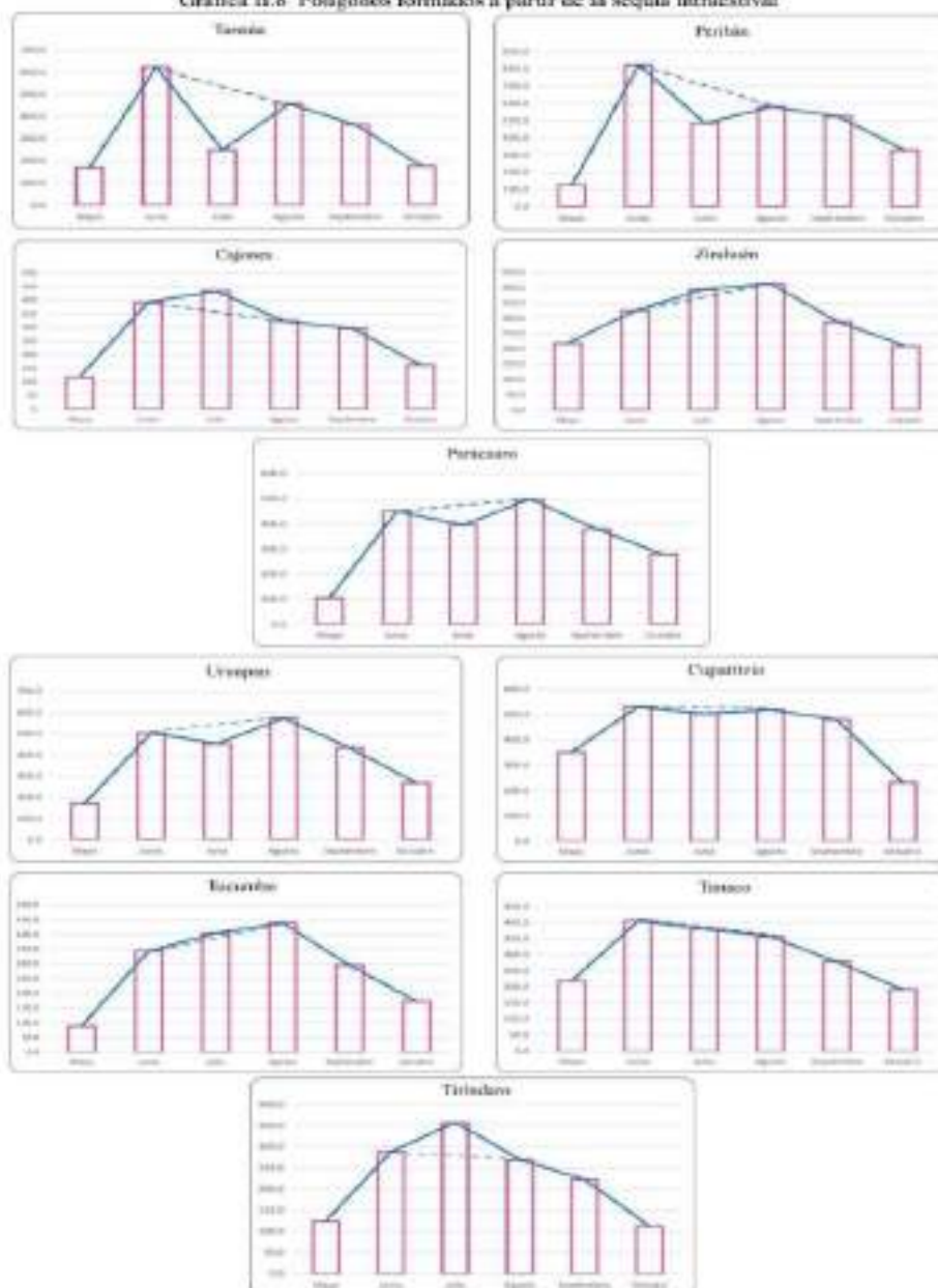
Gráfica II.8. Polígonos formados a partir de la sequía intraestival
