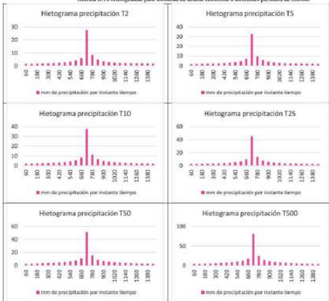
Gráfica II.16 Hietogramas para tormenta de diseño conforme a diferentes periodos de retorno
