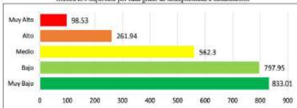
Gráfica II.4 Superficie por cada grado de susceptibilidad a hundimientos
