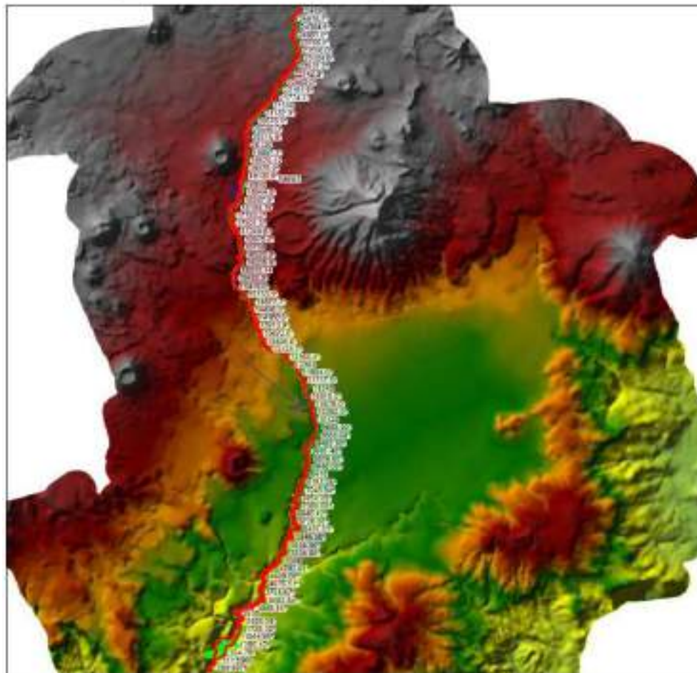
Figura II.54 Superficie de triángulos irregulares y distribución de secciones.
