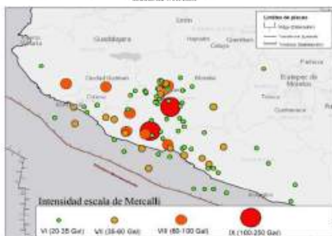
Figura II.15 Localización de sismos que podrían originar aceleraciones suficientes para generar daños de intensidades iguales o mayores a VI en la escala de Mercalli
