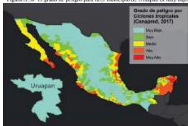
Figura II.30 El grado de peligro para la el municipio de Uruapan es muy bajo
