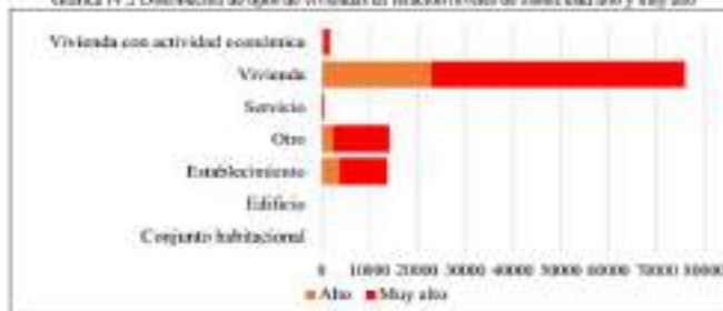
Gráfica IV.2 Distribución de tipos de viviendas en relación a los niveles de sismicidad alto y muy alto
