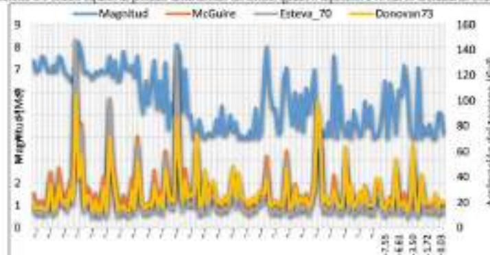
Gráfica II.2 Sismos capaces de producir aceleraciones del terreno iguales o superiores a 16 Gal en la ciudad de Uruapan
