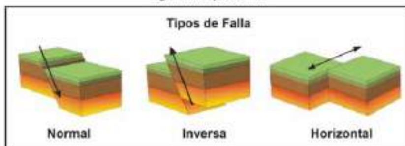
Figura II.18 Tipos de fallas
