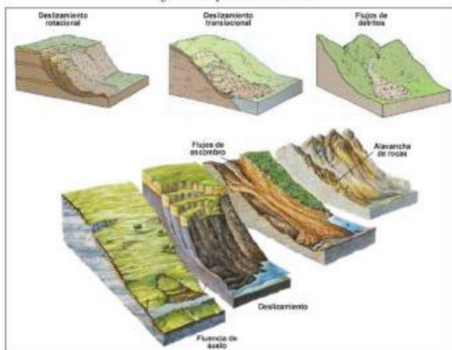
Figura II.16 Tipos de deslizamientos
