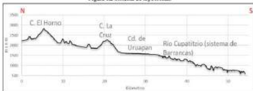
Figura 1.2 Sistema de topoformas
