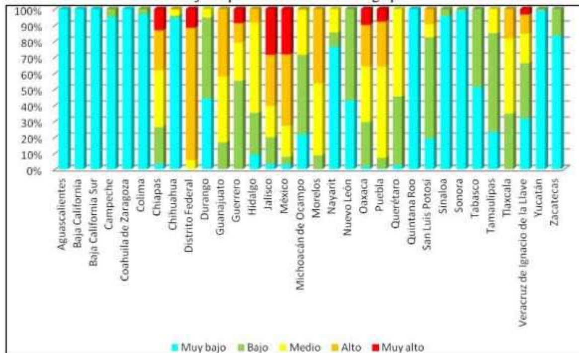
Gráfica II.12 Porcentaje de población estatal en riesgo por tormentas eléctricas
