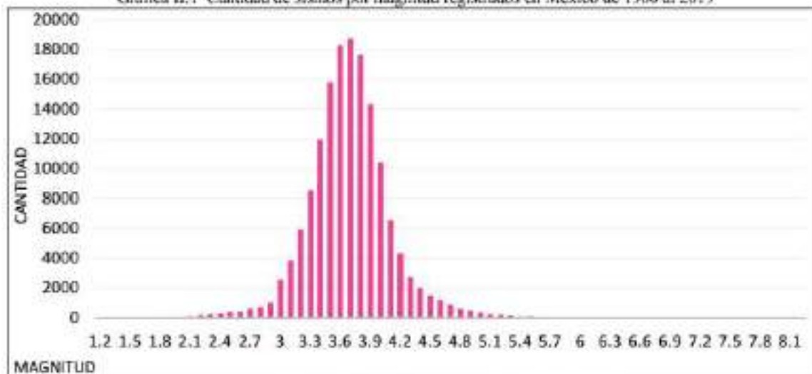
Gráfica II.1 Cantidad de sismos por magnitud registrados en México de 1900 al 2019
