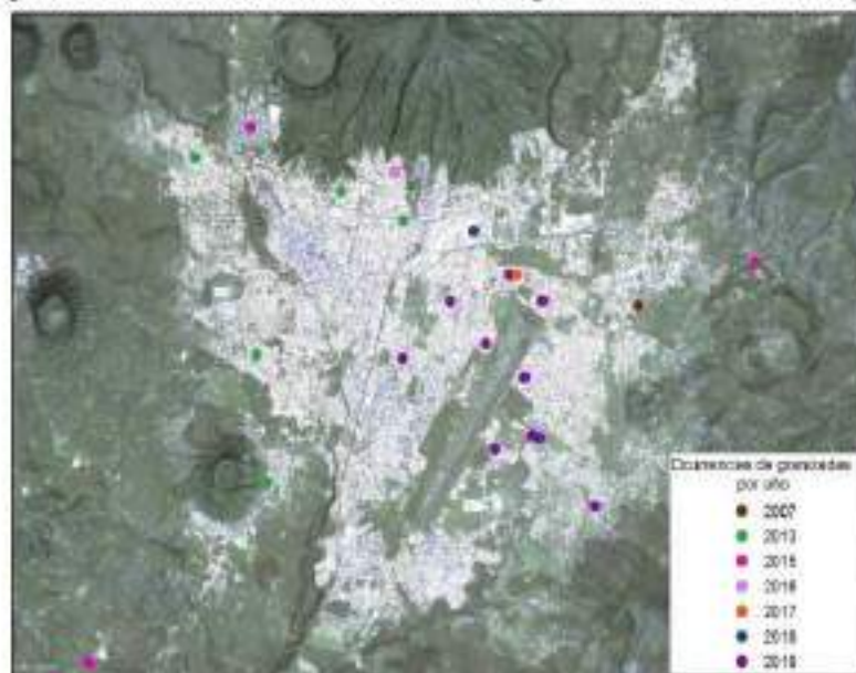
Figura II.25 Distribución de ocurrencias de tormentas de granizo en el área urbana de Uruapan
