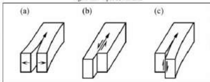
Figura II.19 Tipos de fracturas
