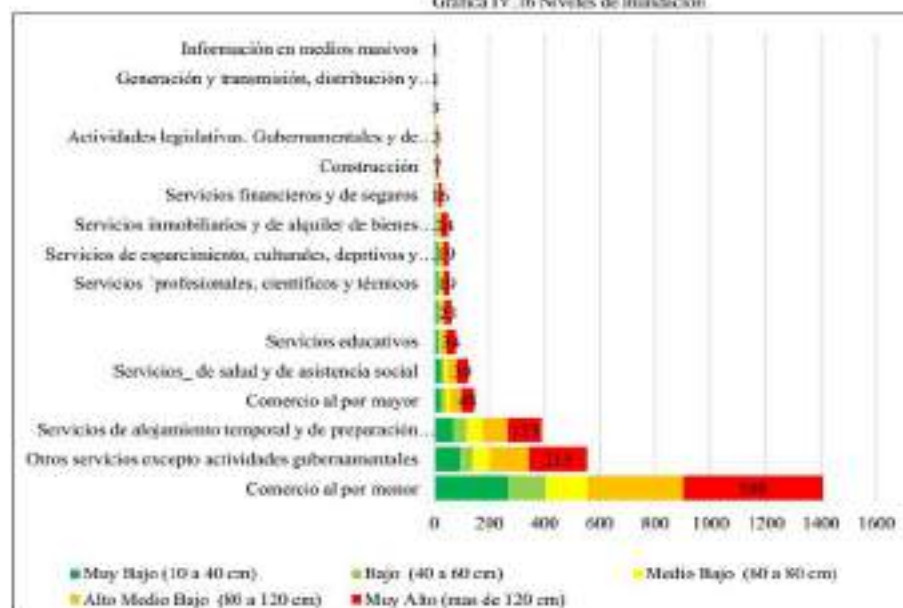
Gráfica IV.16 Niveles de inundación
