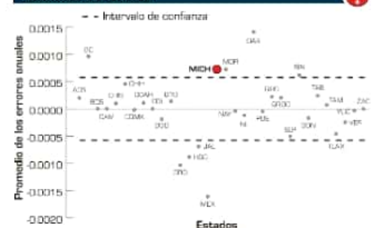
Promedio de los términos de error producidos por las regresiones lineales en cada uno de los estados federativos. Nota: la línea horizontal es el intervalo de confianza a partir de cual los términos de error superan el límite establecido por la distribución estándar.
