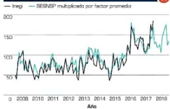
Evolución de los homicidios culposos reportados por el SESNSP y de las denuncias por homicidio publicadas por el Inegi en Michoacán, 2009-2018
